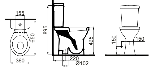
2204-0105 Bedensel Engelli Alttan Çıkışlı Klozet (36x65x49) S-Trap WC Pan
