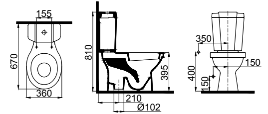
1704-0505 Gökkuşığı Arkadan Çıkışlı Klozet / P-Trap WC Pan (36x67x39) 1704-0105 Gökkuşığı Alttan Çıkışlı Klozet / S-Trap WC Pan (36x67x39)
